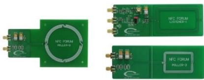
NFCテスト用具セット
